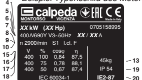
Beispiel Typenschild des Motors
