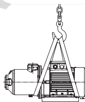
Fig. 7 Sollevamento pompa Raising the pump Anhebung Pumpe Suoilevament de la pompe Elevación de la bomba 吊起水泵
