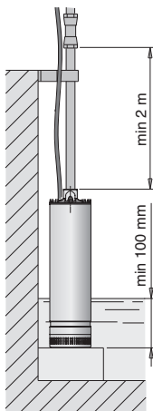
3.93.007/2 Модификация без поплашкового выключателя
