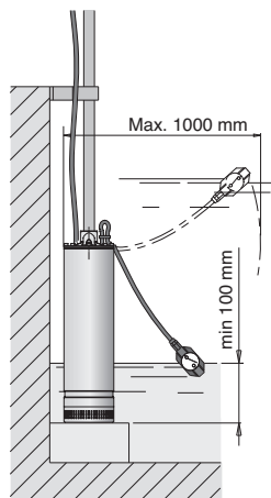
9.93.00712 Ausführung mit Schwimmerschalter
