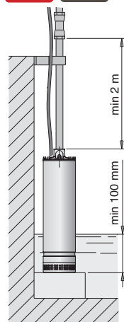
Esecuzione senza galleggiante
