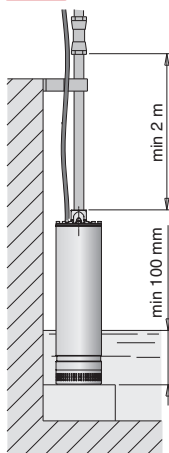
9.93.00712 Ausführung ohne Schwimmerschalter
