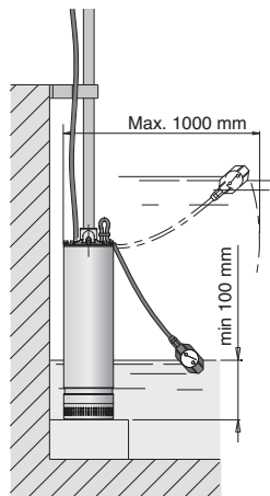
3.93.007/3 Модификация с поплачковым выключателем
