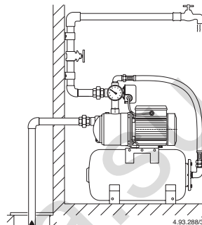
Fig. 2 Funzionamento in aspirazione Suction lift operation Saugbetrieb Fonctionnement en aspiration Funcionamiento en aspiración Sugande funktion Zuigsituatie Θέση λειτουργίας με κάθστη αναρρόφηση Работа выше уровня жидкости 负压水头工作
