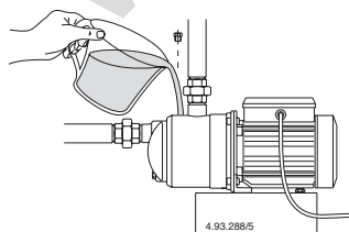
Fig. 4 Riempimento Filling Auffüllung Remplissage Llenado Fyllning Vullen Γέμισμα Наполнение 灌泵
