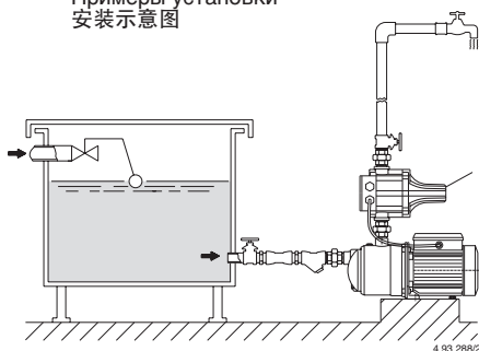
Fig. 1 Funzionamento sotto battente Positive suction head operation Zulaufbetrieb Fonctionnement en charge Funcionamiento bajo carga Tillrinning sugsidan Toelooppositie Θέση λειτουργίας με θετική αναρρόφηση Работа под гидравлическим напором 正吸上水头的操作
