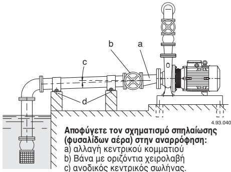
Σχ. 2. Σύνδεση σωληνώσεων
